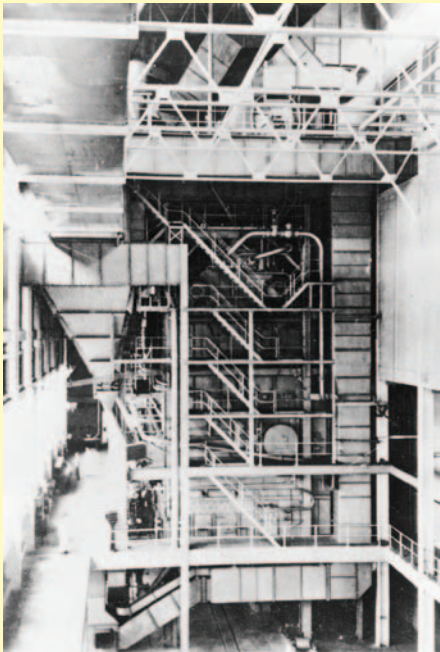
中電發電機組。 (圖片來源：政府新聞處圖片資料)
